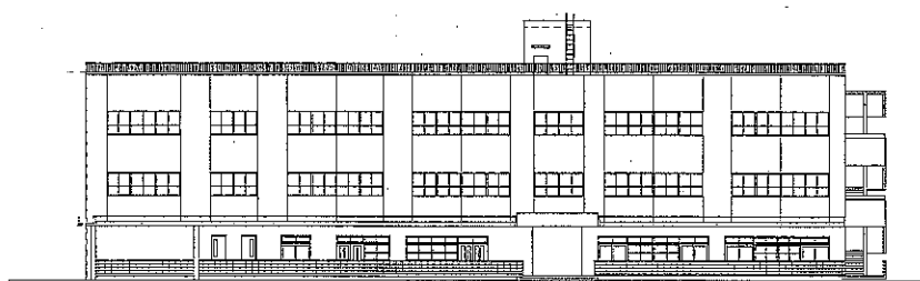
南棟北立面図
