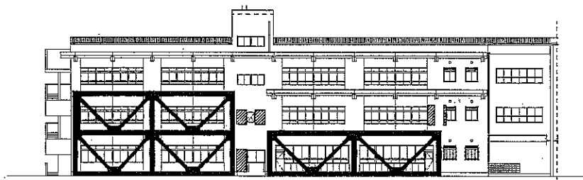
南棟南立面図
