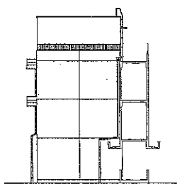
南棟東立面図
