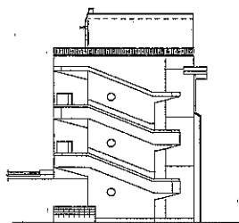
南棟西立面図
