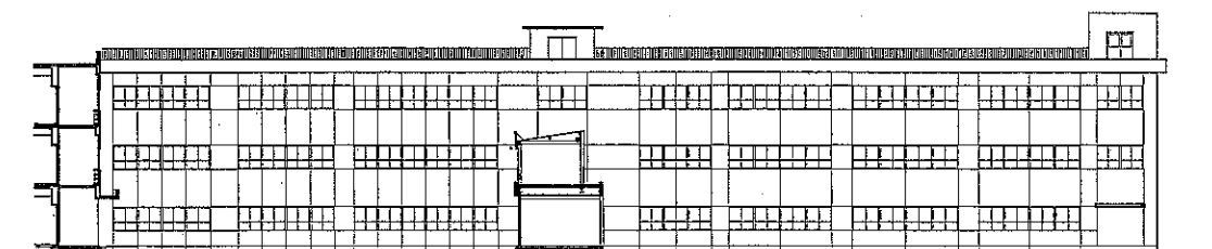
中棟北立面図
