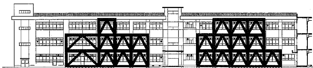
中棟南立面図
