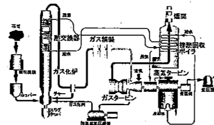
(IGCCの仕組み)
