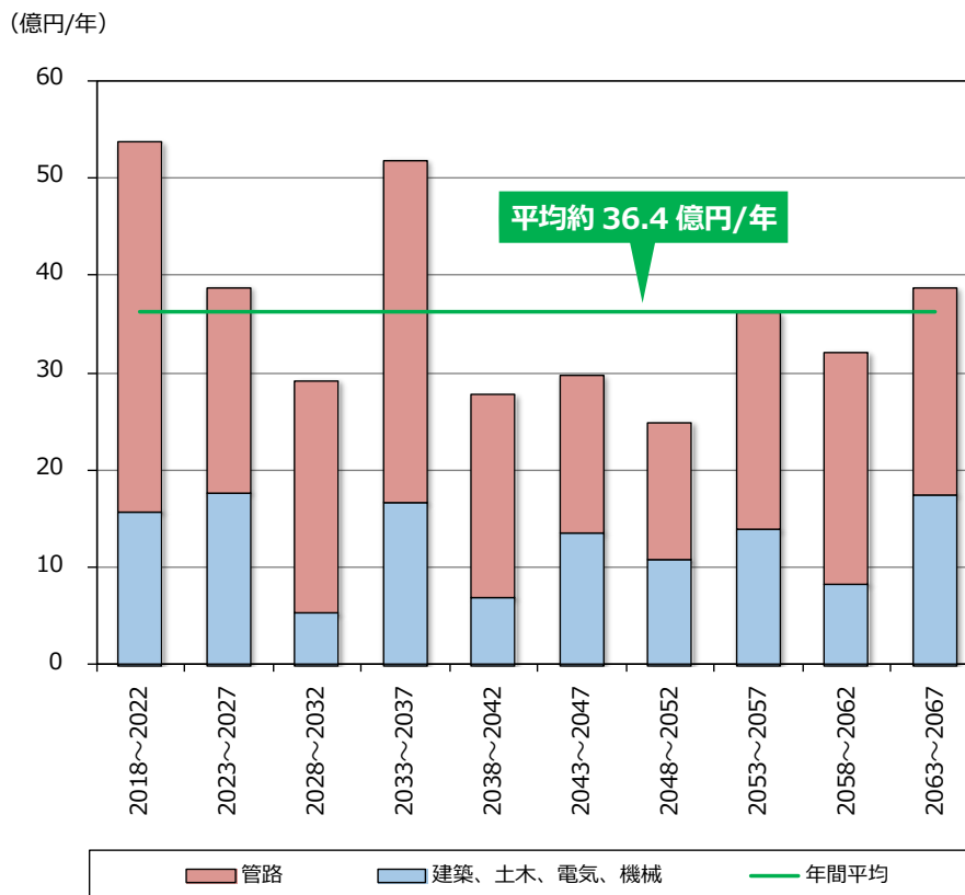
図表 3-4 法定耐用年数で更新した場合の水道施設の更新費用
