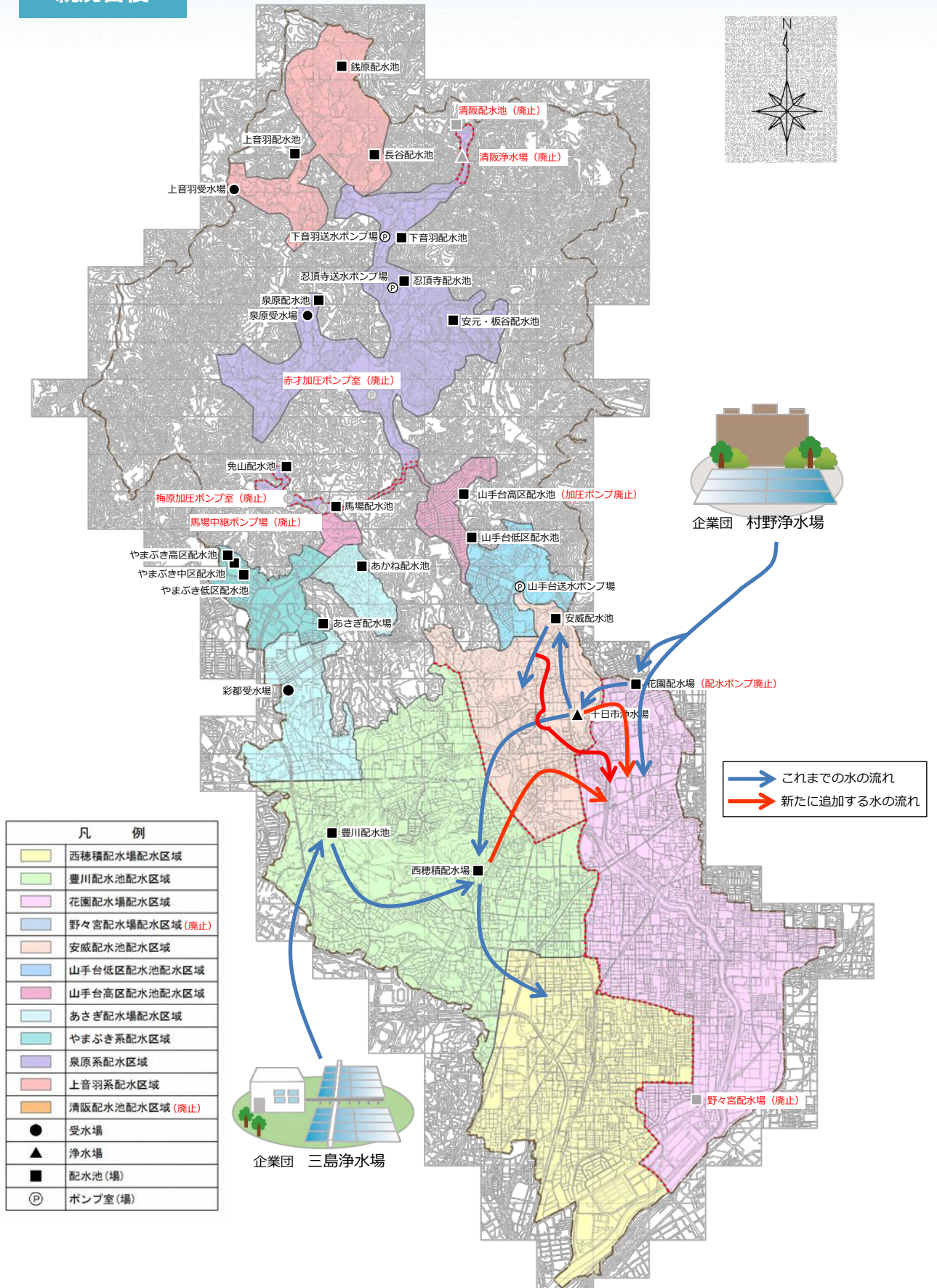
図表 4-7 水道施設位置図 (統廃合後)
