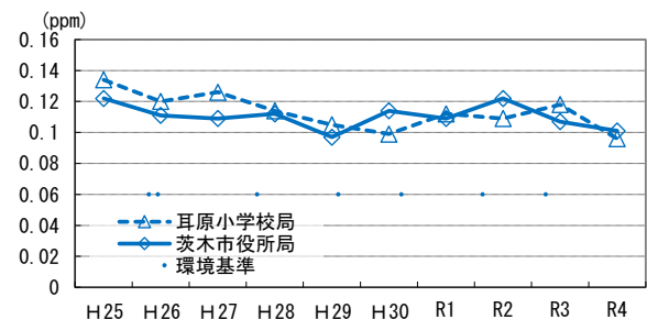
図3 光化学オキシダント (昼間の1時間値の最高値)
