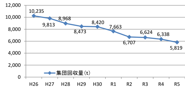
図16 集団回収量
