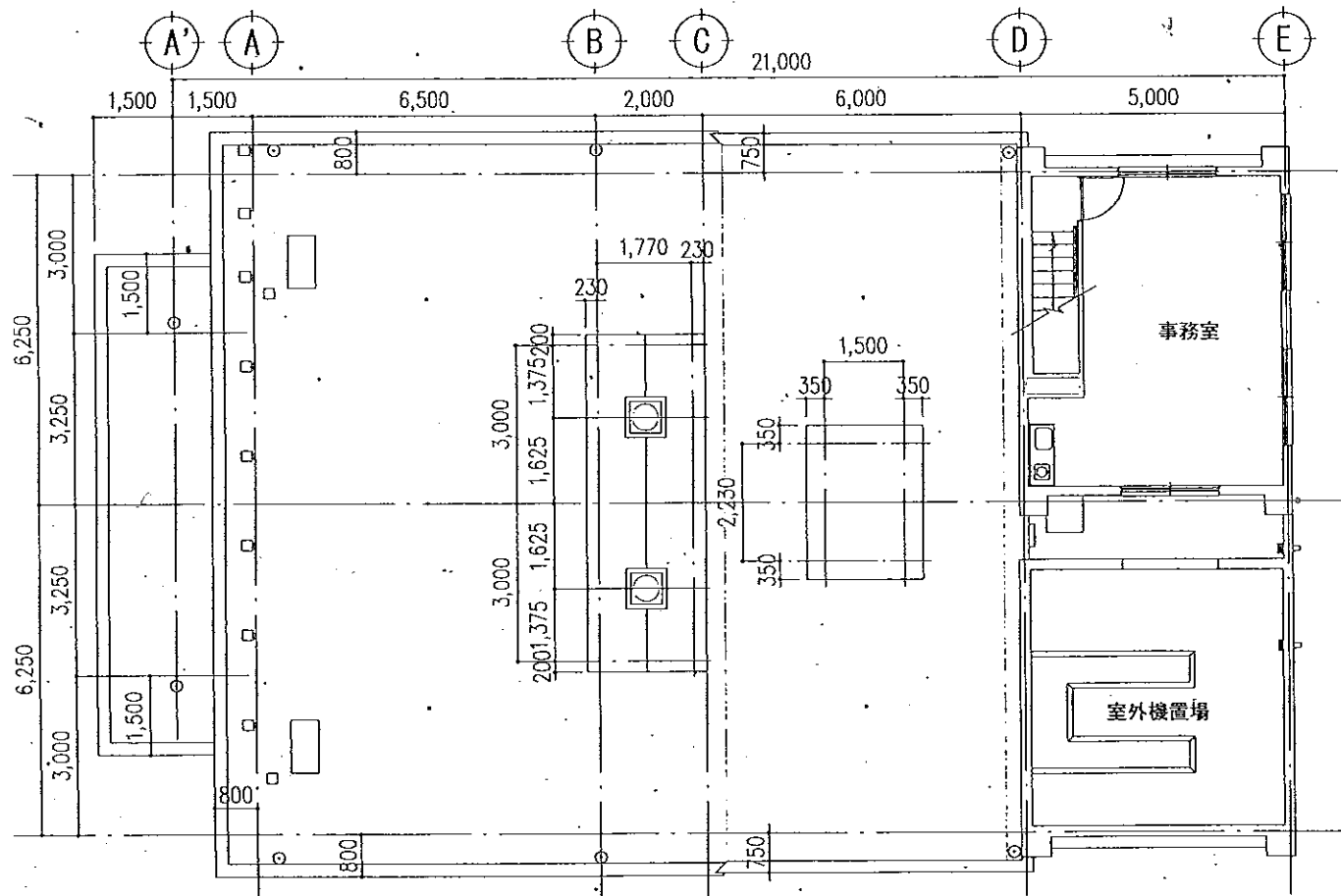
2階平面図 1/100
