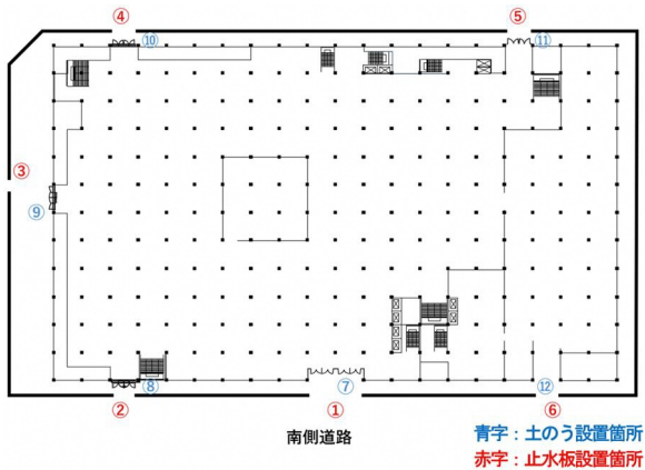
別添 2 浸水防止用設備配置図
