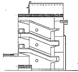
南棟西立面图
