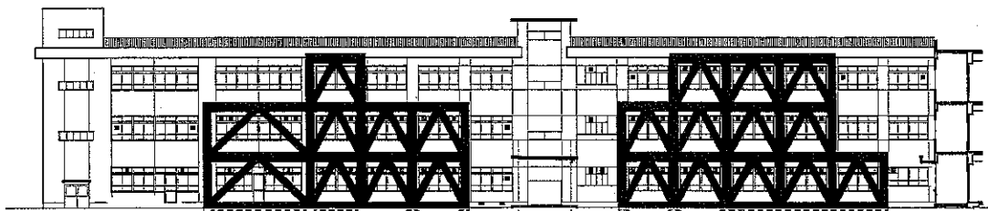
中棟南立面図
