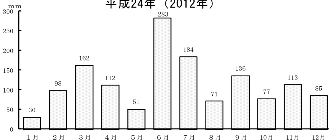
月別降水量（月間値） 平成24年（2012年）
