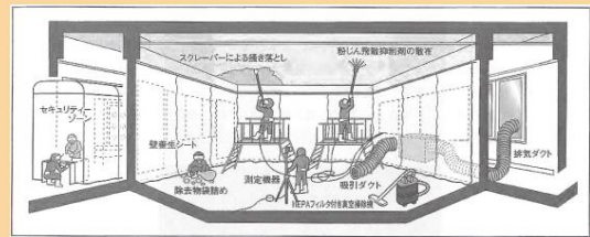
石綿含有吹付け材除去作業概念図
