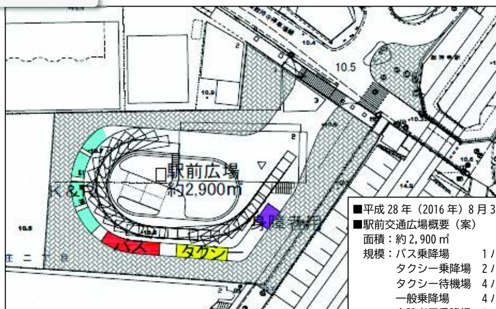
図 駅前広場の整備計画
