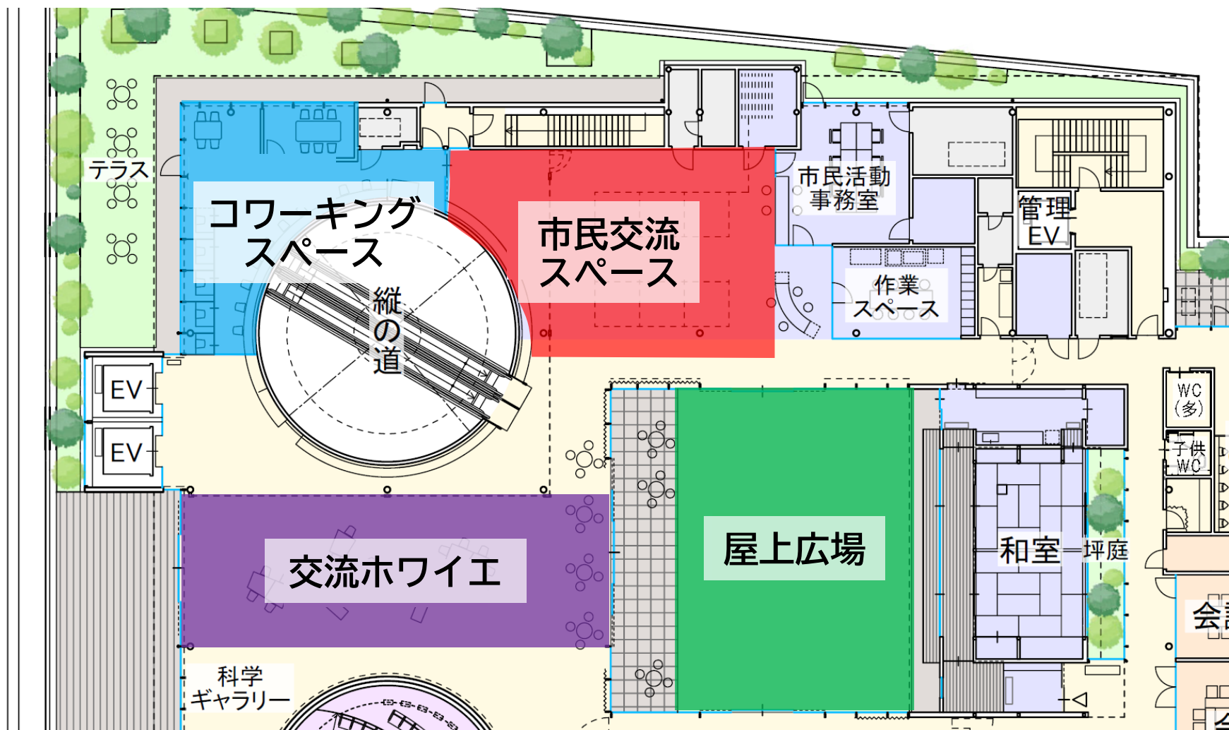
平面図
