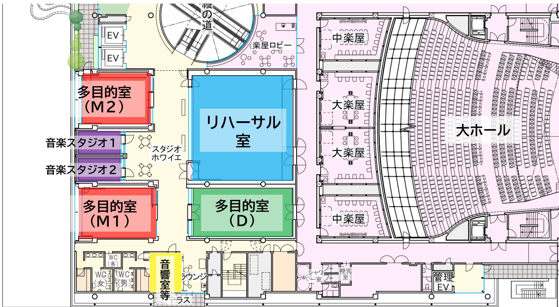
平面図
