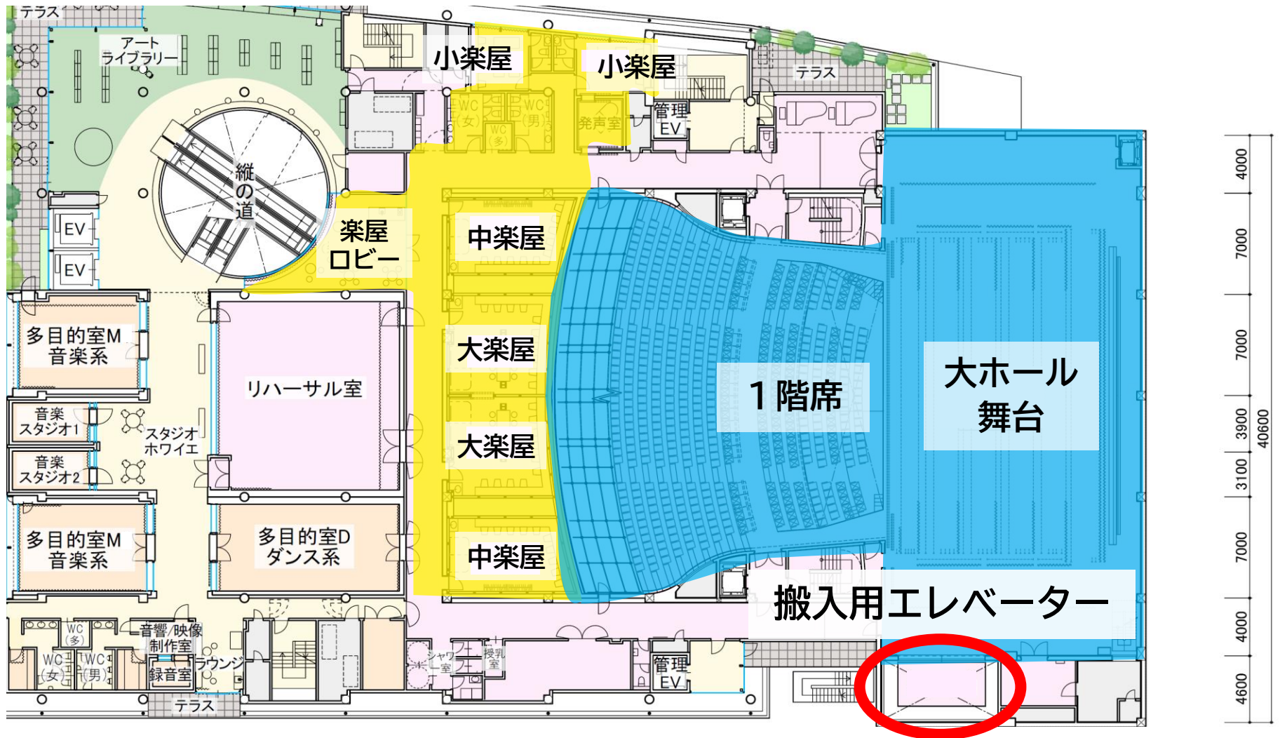
平面図 (3階)
