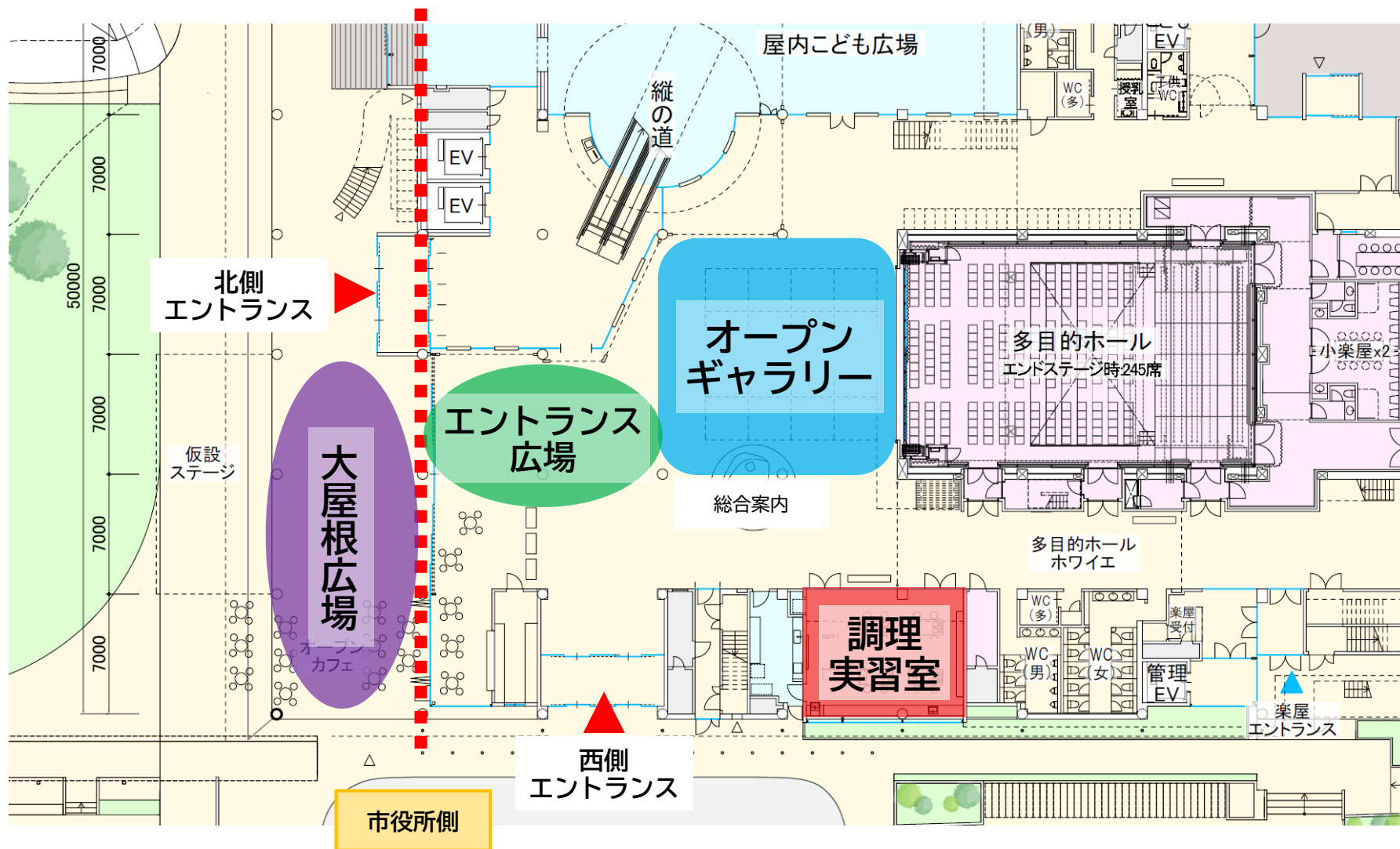
平面図
