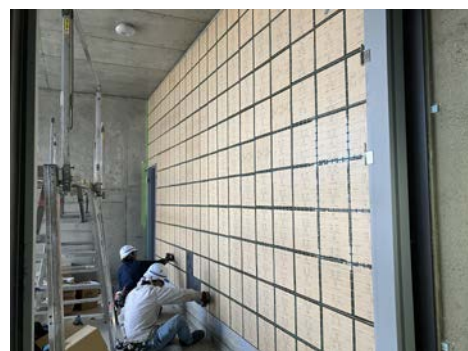
外壁のタイルを張っています。
