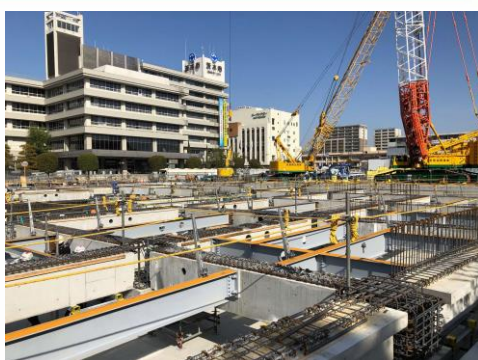
現場で作成したPC梁や鉄骨梁を取付しています。
