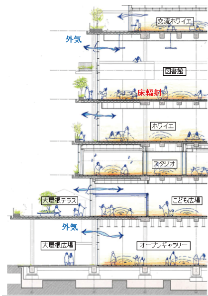
新施設の床輻射のイメージ図
